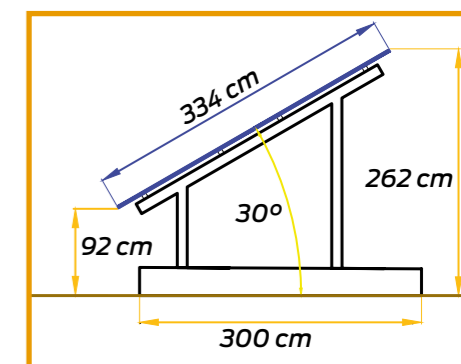
Coupe d'une installation de panneau solaire et ses dimensions.
